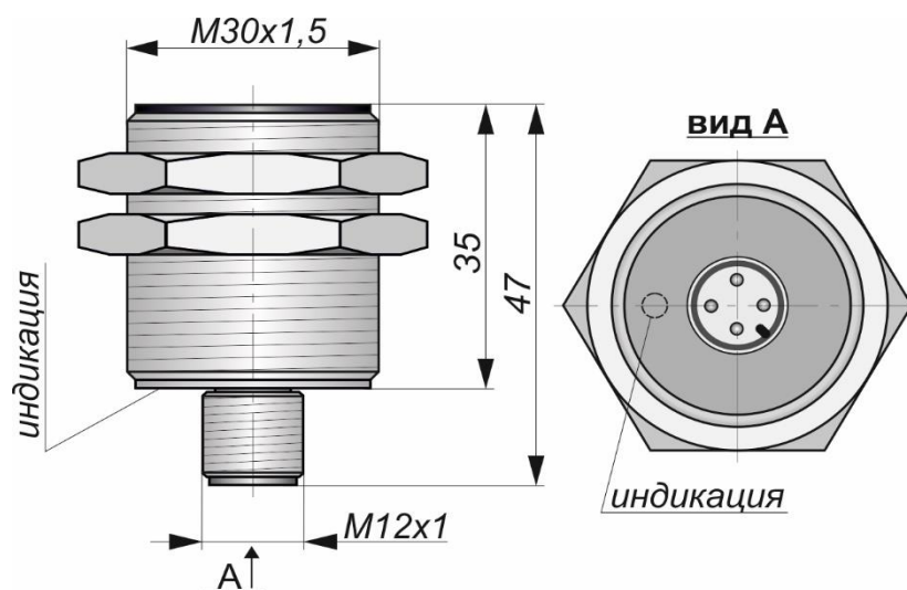
Габаритный чертеж
